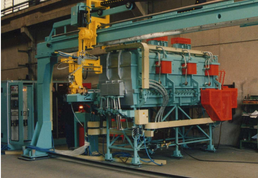
Forno per alluminio
